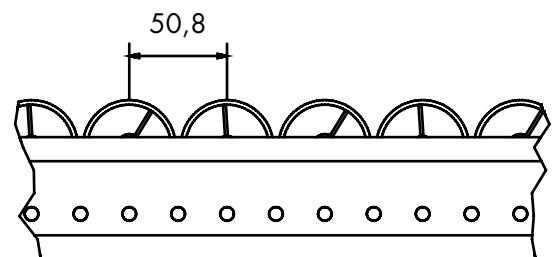
Passo dei rulli
